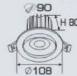
AFC 747 LED 12W 583.000
