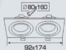
AFC 388/2 T - MR16 (Không Bóng)
